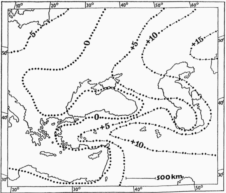
Abb. 3. – Kontinentalitätsstufe von -5-Stufe (Ozeanität) über dem Null-Werte bis zur +15-Stufe in den Räumen der Arealen von Thesium diffusum und T. procumbens und der Nachbarländer (nach Ivanov 1948: Taf. 1).
