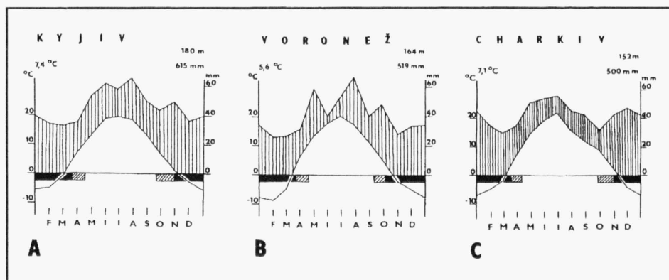
Abb. 2. – Klimadiagramme aus der Nähe einiger Fundorte der Art Thesium diffusum . A – Kyjiv (Kiev), nach Anonymus (1966: 315) und Rudloff (1981: 198). B – Voronež, nach Anonymus (1966: 357). C – Charkiv (Charkov), nach Rudloff (1981: 199).
