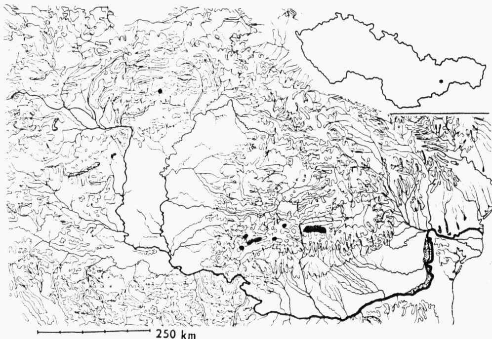
Abb. 3. - Arellen von C. pyrenaica in den Karpaten und Lokalisierung des Fundortes auf dem Trstie-Berge in der Tschechoslowakei.
