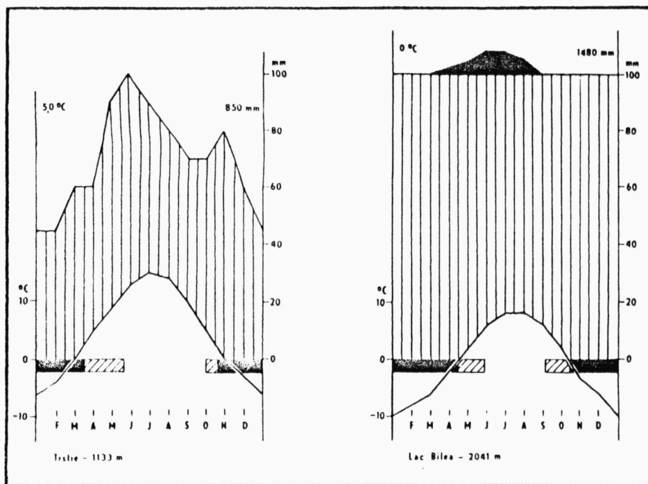
Abb. 2. - Klimadiagramme der Verhältnisse (nach den bezüglichen Karten aus den Klima-Atlanten (Vesecký et al. 1958; Stonescu et al. 1966) zusammengestellt) im Gipfelabschnitt des Trstie-Berges und der Umgebung des Gebirgsees Lac Bilea, nördlich des Capra-Berges (2405) im Mittelabschnitt des Gebirges Muntii Fagarasului, einen von den Fundorten C. pyrenaica in den Südkarpaten.
