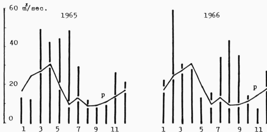
Obr. 2. - Průměrné měsíční průtoky Divoké Orlice u Týniště n. Or. (m /sec.) v letech 1965 a 1966 a jejich porovnání s dvacetiletým průměrem 1943-1962 (p).
