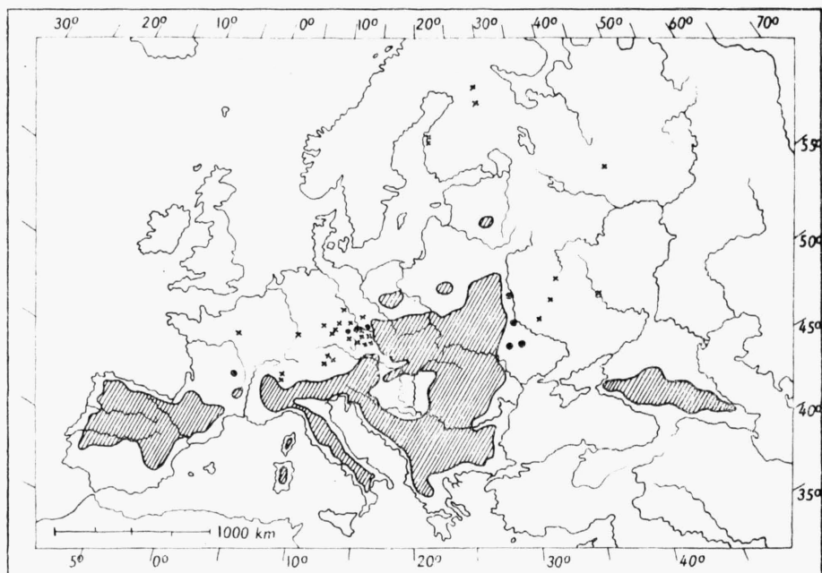
Fig. 2. — Das europäische und kaukasische Subareal von Cruciata glabra einschliesslich der offensichtlich sekundären, mit Kreuzen bezeichneten Lokalitäten.
