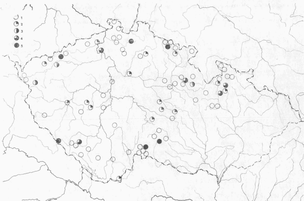
Abb. 1. — Verbreitung von Botrychium matricariifolium in der ČSR. — 1 — Literaturangaben 2—5 — Untersuchte Herbarbelege nach den Sammlungsjahren: 2 — vor dem Jahr 1900. 3 — 1900 bis 1925. 5 — 1926—1945. 6 — 1946—1975.
