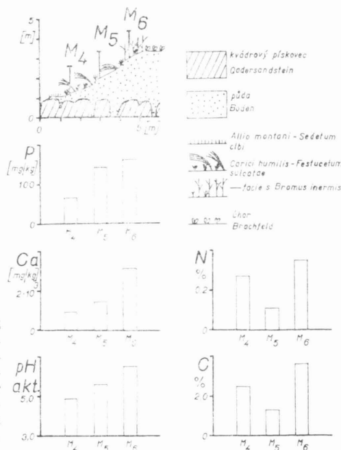
Obr. 2. — Rozdílnost chemismu půdy z měříšť umístěných na spádnicí svahu na lokalitě u Mnichova Hradiště, v asociaci Carici humilis-Festucetum sulcatae KLIKA 1951. — Abb. 2. — Verschiedenheit des Bodenchemismus der an der Abhangslinie befindlichen Messstellen an der Lokalität bei Mnichovo Hradiště in der Assoziation Carici humilis-Festucetum sulcatae KLIKA 1951.
