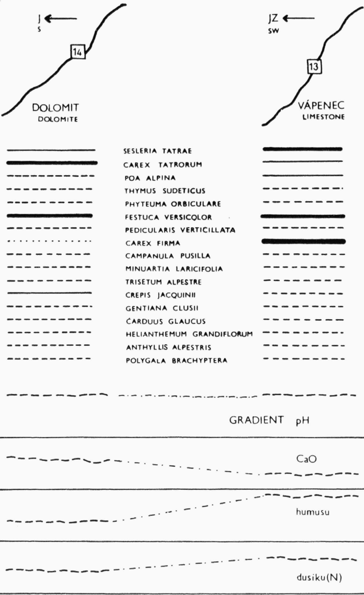
Obr. 5. — Vegetační a ekologické poměry na vápenci a dolomitu na prudkých svazích k J a JZ mezi Velkým Krivánem a Pekelníkem 1580 až 1650 m n. m. Další popis viz obr. 2. — Fig. 5. — Vegetational and ecological conditions on limestone and dolomite on steep S and SW slopes between Velký Kriván and Pekelník, 1580 to 1650 m above sea level. Further description see fig. 2.
