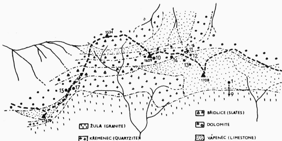
Obr. 1. — Mapa hřebenu Kriváňské Malé Fatry od Velkého Kriváně (1708 m) přes Pekelník (1609 m), Koniarky (1534 m) k Malému Krivání (1670 m) s přibližným vyznačením geologických poměrů a lokalit odebraných vzorníků 1 až 17. — Fig. 1. — A map of the crest of the Kriváňské Malá Fatra Mts. from Velký Kriváň (1708 m), Pekelník (1609 m) and Koniarky (1534 m) to Malý Kriváň (1670 m) with geological layers and localities of studied samples 1 to 17.
