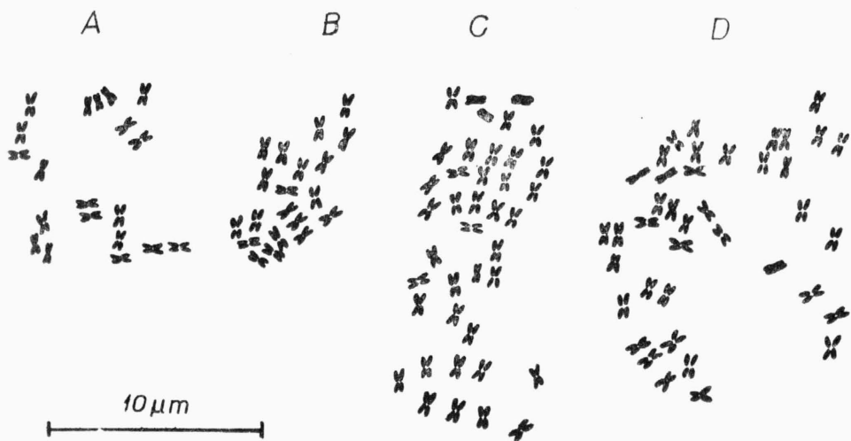
Abb. 1. — Metaphaseplatten somatischer Zellen. — A: Anagallis parviflora HOFFMANNS. et LINK., 2n = 20 ; B: A. linifolia L., 2n = 20 ; C: A. arvensis L., 2n = 40 ; D: A. foemina MILL., 2n = 40 .
