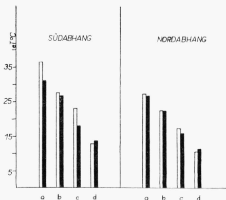
Abb. 2. — Vergleich der durchschnittlichen Exponentialtemperatur auf zwei Expositionen auf Spilithängen (weiss) und auf Schieferhängen (schwarz); a — Frühjahr (vom 1. April—21. Juni), b — Frühsommer (vom 21. Juni—10. August), c — Spätsommer (vom 10. August—3. November), d — Herbst und Winter (vom 3. November—12. April).
