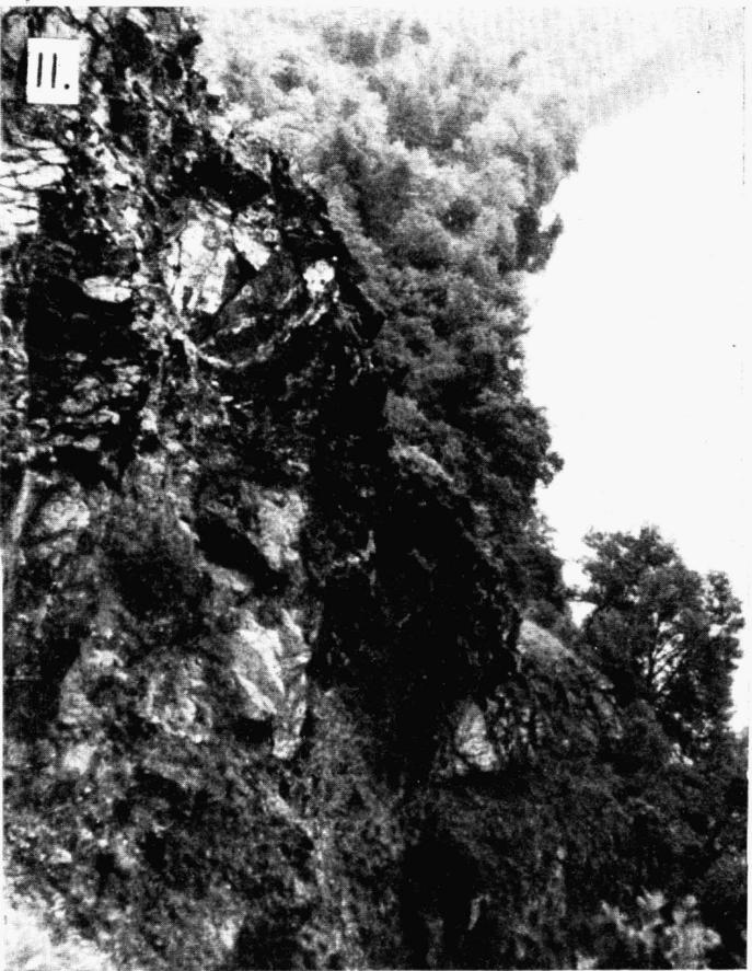
II.: Spilitfelsvorsprünge mit Pioniergeellschaften.
