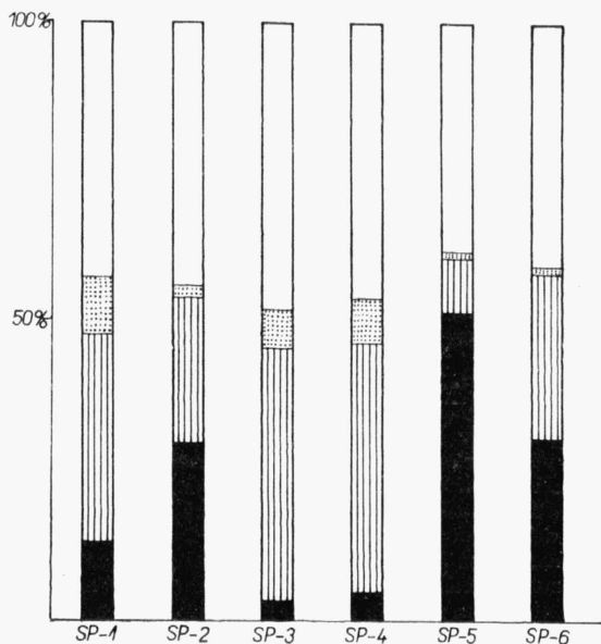
Abb. 7. — Vergleich der Anteile: Mineralteilen (schwarz), Humus (schraffiert), organischer Relikte (punktiert), und Bodenhohlräume (weiss) auf verschiedenen Standorten der Spilite: Südhang (SP-1), Südhang unter dem Gipfel (SP-2), Gipfel (SP-3), Nordhang (SP-4), Steinhalde (SP-5), Nordwesthang (SP-6).
