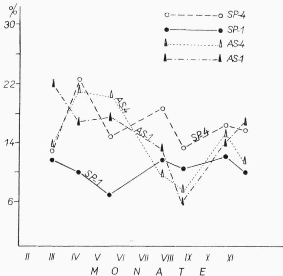
Abb. 5. — Veränderungen des Wassergehaltes des Bodens im Laufe des Jahres 1966 auf Spiliten und algonkischem Schiefer; (SP-1) — Südhang des Spilitfelsens, (SP-4) — Nordhang des Spilitfelsens, (AS-1) — Südhang des Schieferfelsens, (AS-4) — Nordhang des Schieferfelsens.
