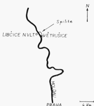
Abb. 1. — Geographische Lage der Spilitzone mit den Versuchsfächen im Moldautal nördlich von Prag.
