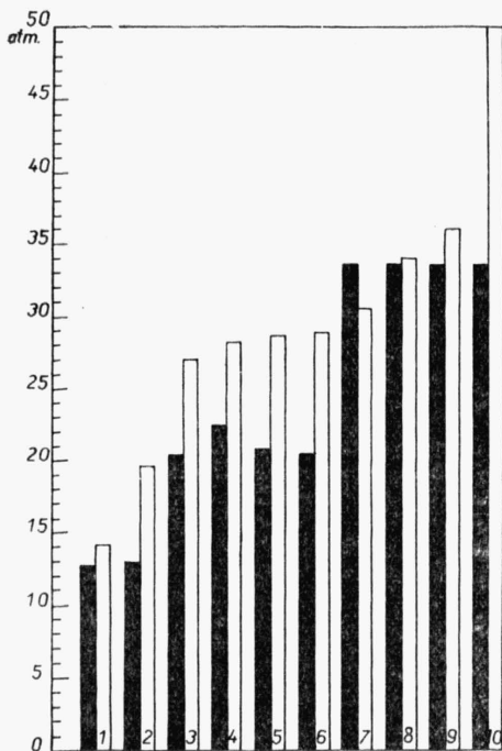
Abb. 3. — Maximale Wurzelsaugkraft von Kräuterarten und Wurzelsaugkraft der Esche, die gemeinsam am selben Standorte wachsen. Schwarz: Wurzelsaugkraft der Esche. Weiss: 1. Aegopodium podagraria , 2. Mercurialis perennis , 3. Geum urbanum , 4. Fragaria vesca , 5. Carex muricata ssp. contigua , 6. Lamium maculatum , 7. Viscaria vulgaris , 8. Sanguisorba minor , 9. Cynanchum vincetoxicum , 10. Calamintha clinopodium
