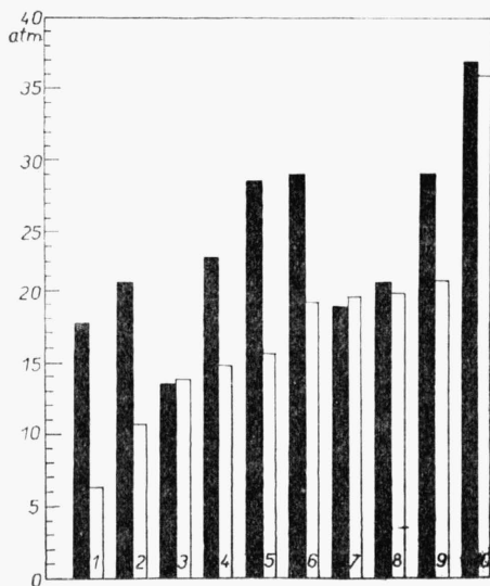
Abb. 1. — Maximale Wurzelsaugkraft einer mesophilen Kräuterart und Wurzelsaugkraft der Esche, die gemeinsam in einem Gefäß wuchsen. Schwarz: Wurzelsaugkraft der Esche. Weiss: 1. Milium effusum , 2. Asarum europaeum , 3. Lamium galeobdolon , 4. Aegopodium podagraria , 5. Viola riviniana , 6. Hepatica nobilis , 7. Mercurialis perennis , 8. Stellaria holostea , 9. Pulmonaria officinalis , 10. Poa trivialis
