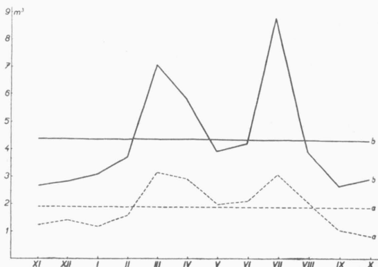
Abb. 2. — Die Abflussverhältnisse des Blanice-Flusses: Die mittleren monatlichen Abflussmengen in m^3/s in dem Zeitraume der Jahre 1951—1960. — a: Pegel Podedvory, b: Pegel Heřmaň (s. Längsprofil des Flusses).
