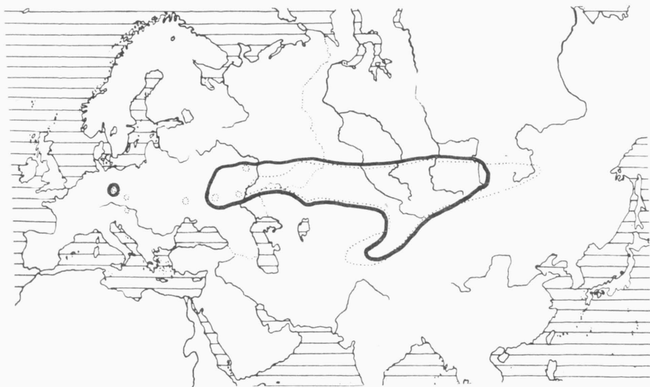
Abb. 5. — Skizze des Areals von Stipa rubens P. SMIRN. s. ampl. und von Helictotrichon desertorum (LESS.) NEVSKIJ. [Areal der letztgenannten Art punktiert und nach GAJEVSKI (1934) und HOLUB (1962) gezeichnet.]
