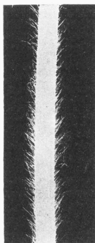
Abb. 4. — Stipa dasyphylla ČERN., Oblik, ein Teil des Grundblattes.
