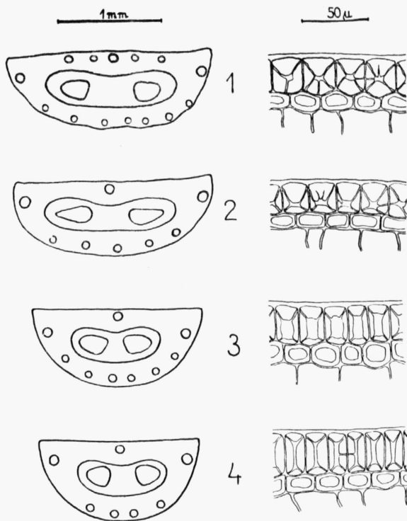
Obr. 5. Schéma příčného řezu jehlicí a příčný řez pokožkou jehlice: 1. Pinus silvestris L., 2. Mlýňanský strom, 3. Pinus digenea BECK, 4. P. mugo ssp. uncinata var. rotundata (LINK) DOM. Zvětšení udáno.
