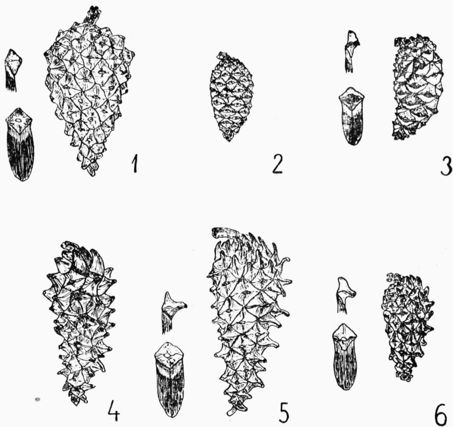
Obr. 4. Typy šišek: 1. Pinus silvestris L., 2. P. digenea BECK, 3. P. mugo ssp. uncinata var. rotundata (LINK)DOM., 4. P. silvestris var. hamata WILLK., 5. Mlyňanský strom, 6. P. mugo ssp. uncinata var. rostrata (ANT.)DOM. Dvě třetiny skutečné velikosti.
