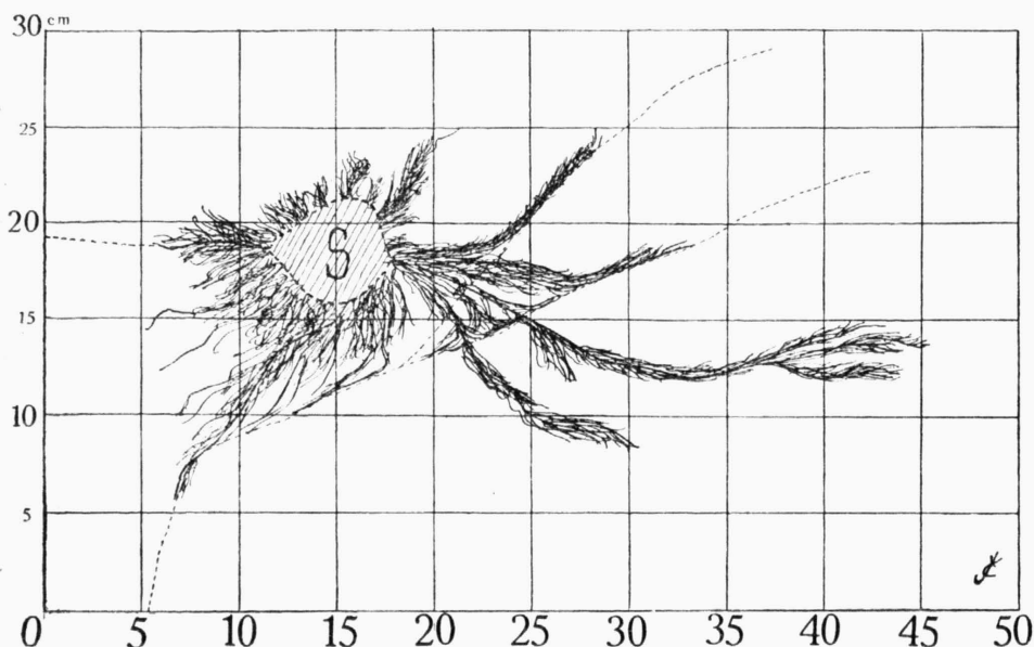
Obr. 2. Kořenový systém žebrovice různolisté jako chasmoexochoomofyta na skalní stěně v Divoké soutěsce (Labské pískovcové pohoří). Vyčárkováná ploška značí ústí dutiny, asi 5 až 7 cm hluboké, v níž byl oddenek a masa kořenů (označeno písmenem S). Oddenek s kořeny hustě vyplňovaly celou dutinu. Na obrázku jsou odstraněny listy a vykreslen kořenový systém, prostírající se po okolní svislé skalní stěně pod povlakem bryofyt. Čárkované linie značí drobné nerovnosti (nepatrné praskliny a lištičky) na povrchu skalní plochy. Orig. J. Čeřovský 1952—53.
