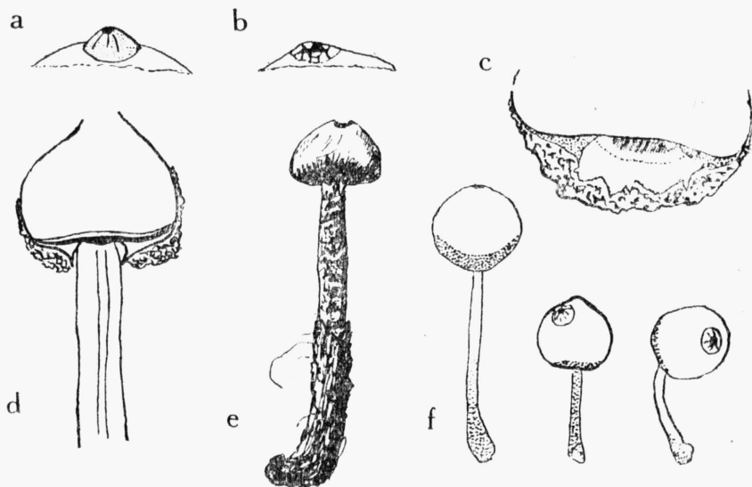
Obr. 1. a) T. fimbriatum sensu H o l l ó s — ústí — mouth — устье. b) T. granulosum L é v. — ústí — mouth — устье. c) T. hollosii M o r. — řez plodnice s vyloženým třením — section without a stem. d) T. hollosii M o r. — řez celou plodnicí — section of receptacle. e) T. fimbriatum Fr. f) T. fimbriatum sensu H o l l ó s (a, b, f, ex H o l l ó s, e — ex Th. C. E. Fries, c, d — orig.)
