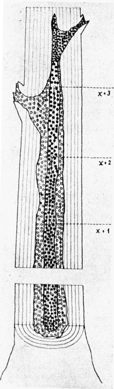
Obr. 7. Schema vzniku složeného jádra. (Orig.) (Vlevo.)
